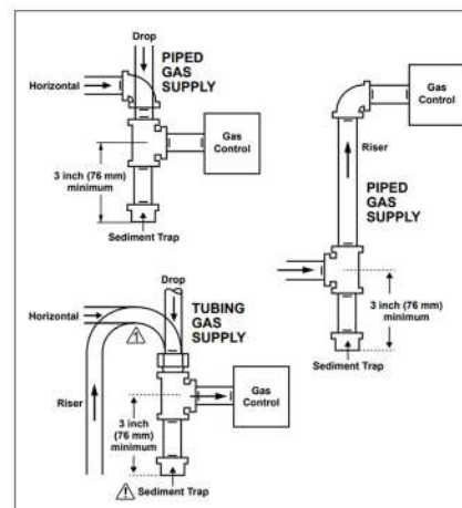
Sediment Trap
