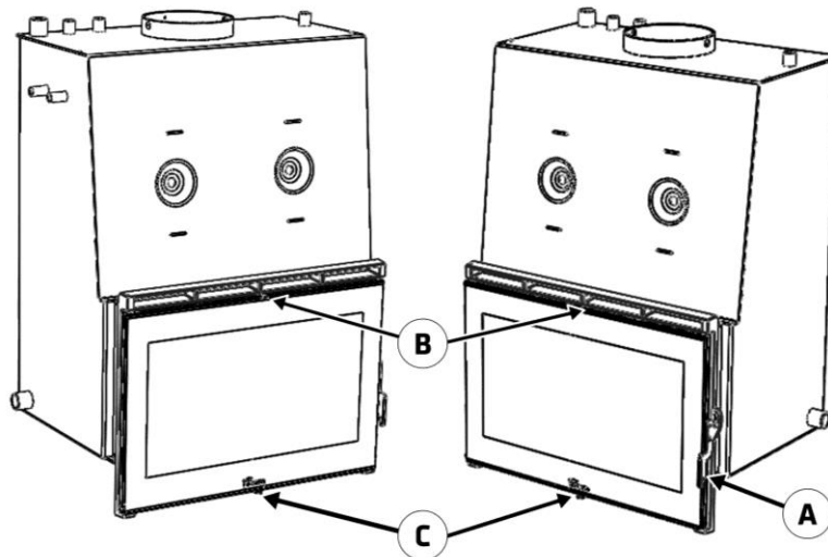
Figura nº15 - Elementos de funcionamiento del aparato
