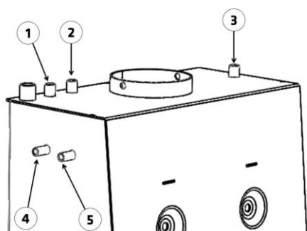
Figura nº13 - Racores de conexión en la pila
