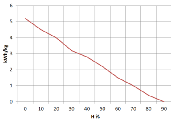
Figura nº14 - Relación entre humedad y poder calorífico de la leña.
