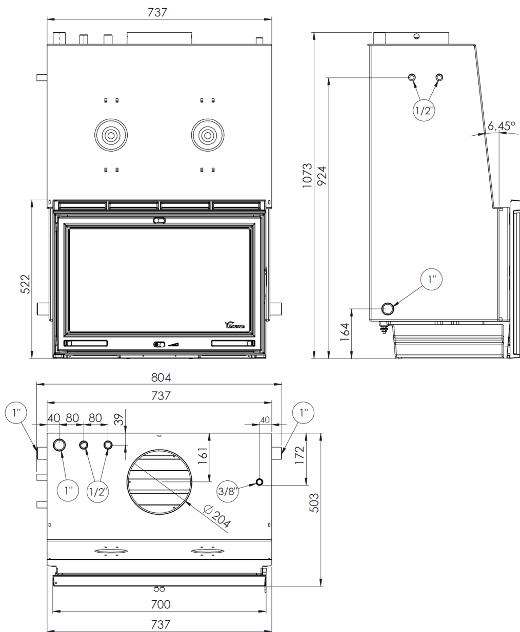
Figura n°1- Dimensiones en mm del aparato SARRIA 20 - SAKAN 20
